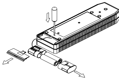
Рис.5. Способ вскрытия ячейки для элементов питания
